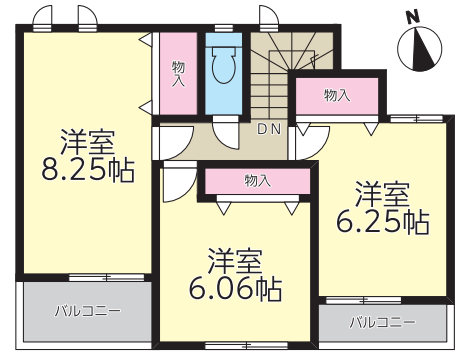
2階平面図:45.55㎡(13.77坪)
